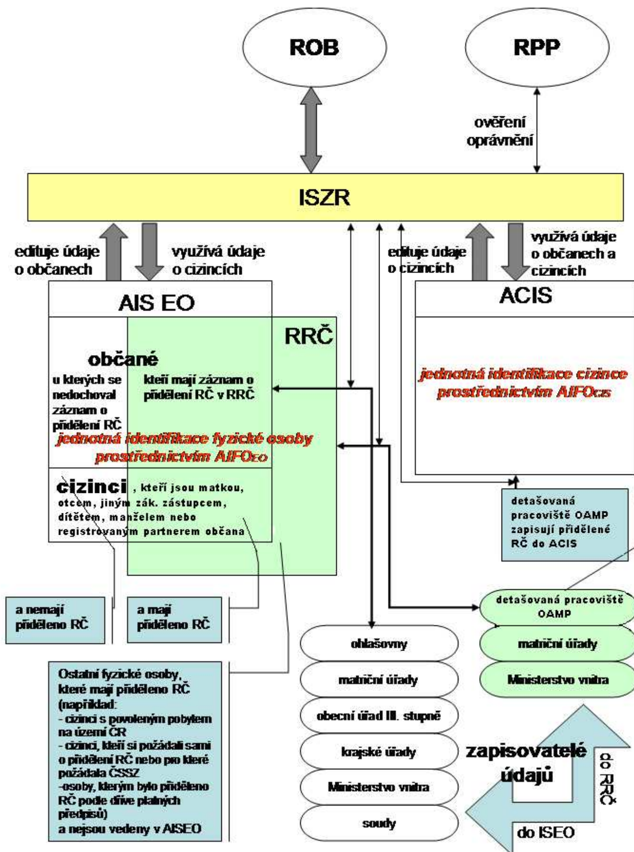
Obrázek: Propojení registru s informačním systémem evidence obyvatel v zjednodušeném kontextu základních registrů
